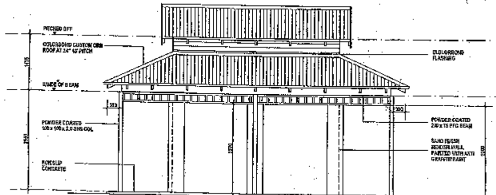
ELEVATION 2
