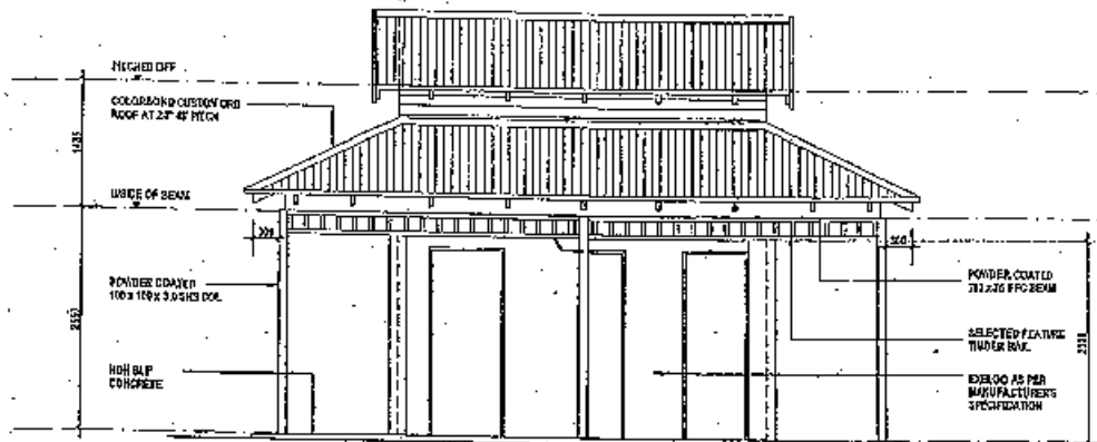
ELEVATION 1
